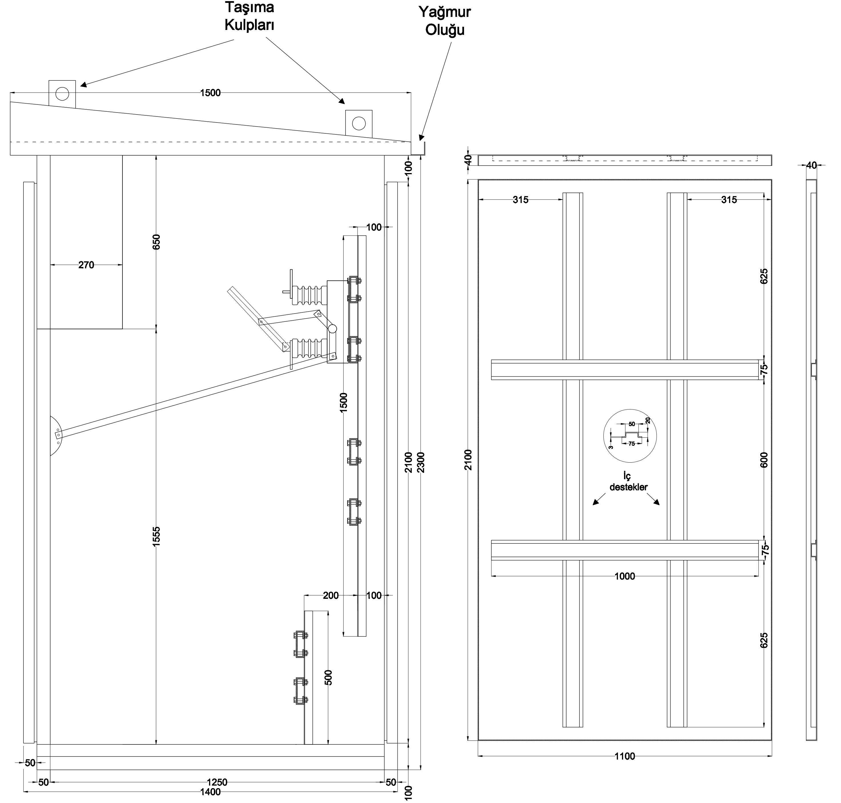
AYIRICI MONTELİ YAN GÖRÜNÜŞ
