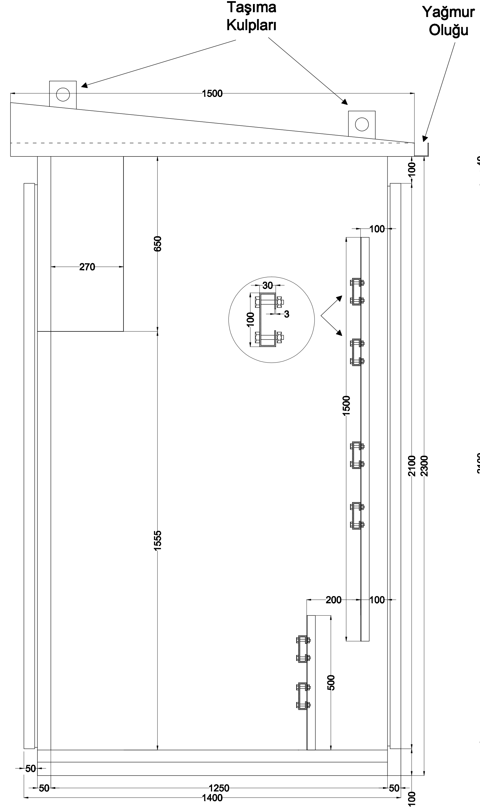
KAPAKSIZ YAN GÖRÜNÜŞ
