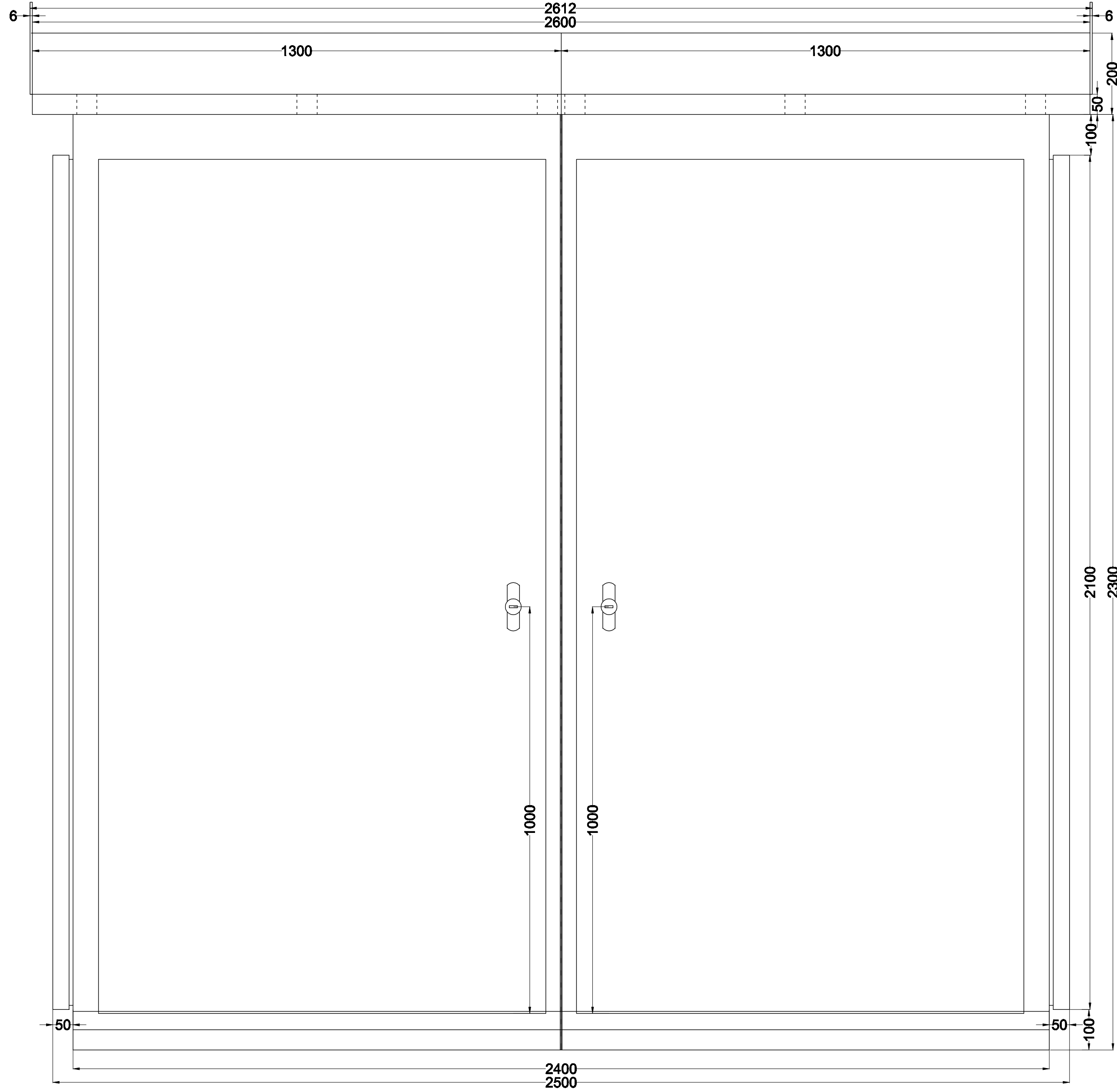
KAPAKLI ÖN GÖRÜNÜŞ
