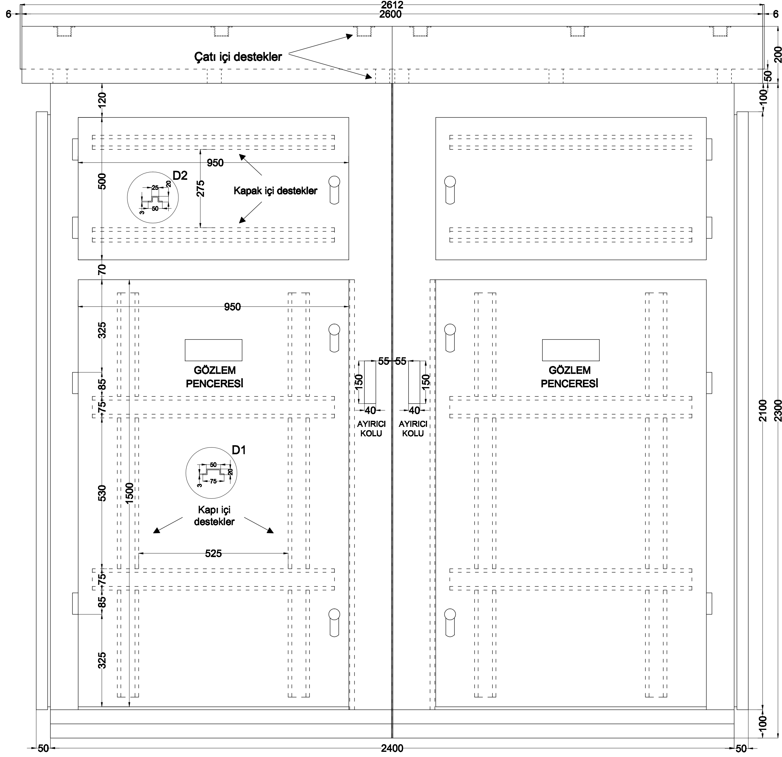
İÇ KAPAKLI ÖN GÖRÜNÜŞ ve İÇ KAPAK DETAY GÖRÜNÜM
