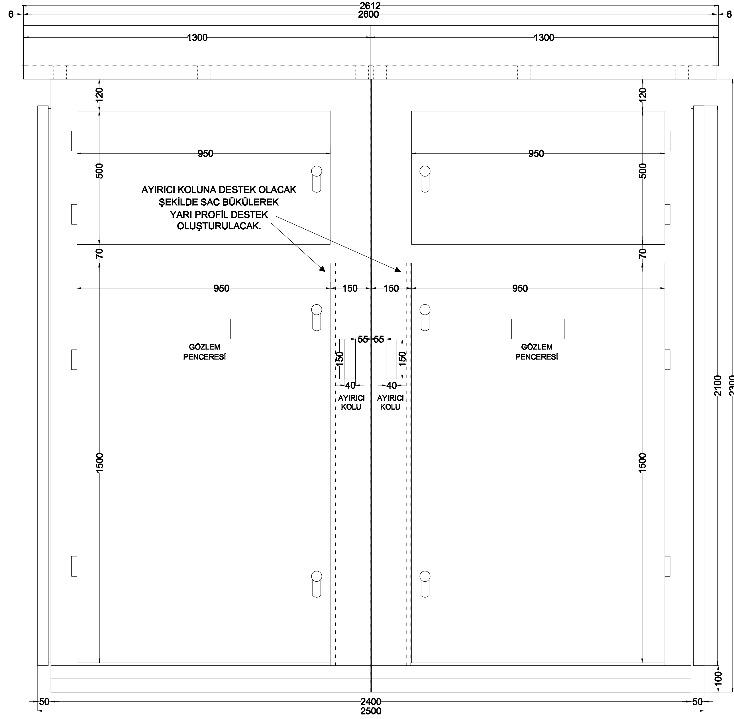
İÇ KAPAKLI ÖN GÖRÜNÜŞ
