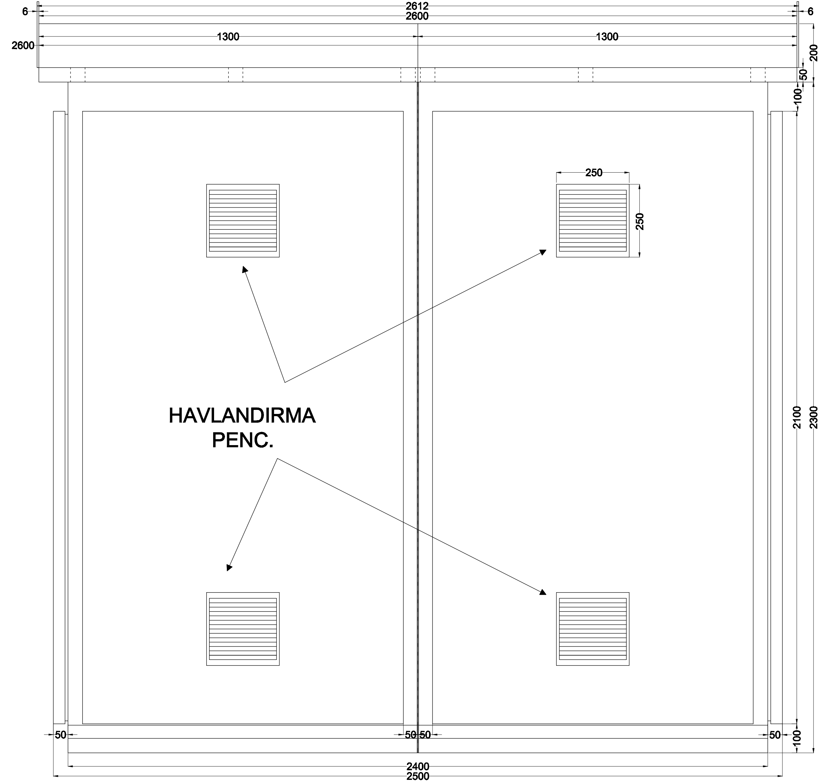
KAPAKLI ARKA GÖRÜNÜŞ
