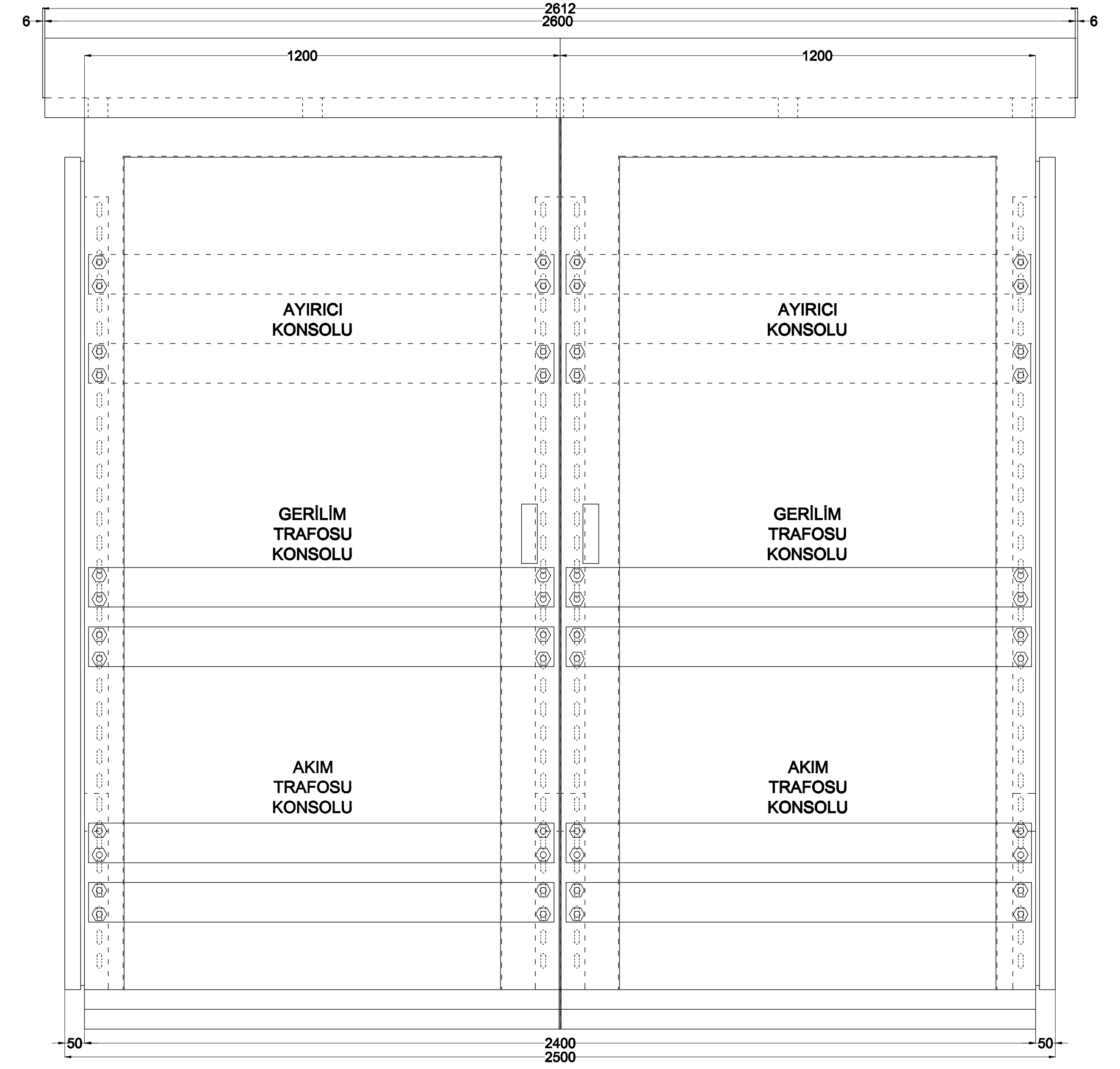
İÇ KAPAKSIZ ÖN GÖRÜNÜŞ
